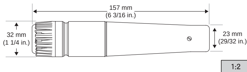
OVERALL DIMENSIONS - DIMENSIONS HORS TOUT
