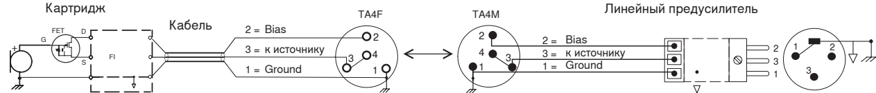
монтажная схема
