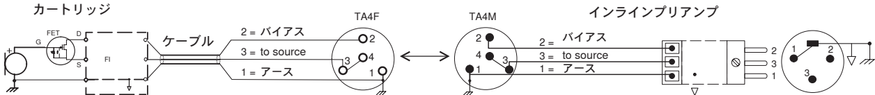
配線図
