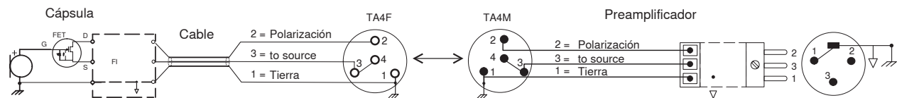
Diagrama de alambrado
