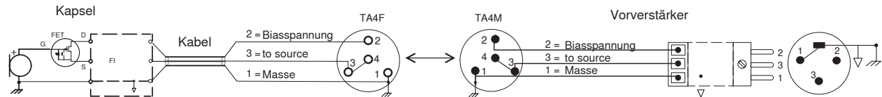
Anschlussplan
